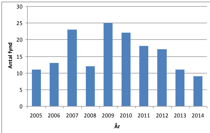
Figur 1. Antal fynd av mindre hackspett 2005-2014
